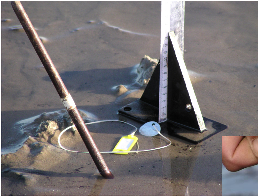
Foto 4. Meetlineaal met meetvoet. Deze wordt steeds op dezelfde wijze op de bodem gezet waarna de lengte van het meettouw langs de schaal wordt afgelezen.
