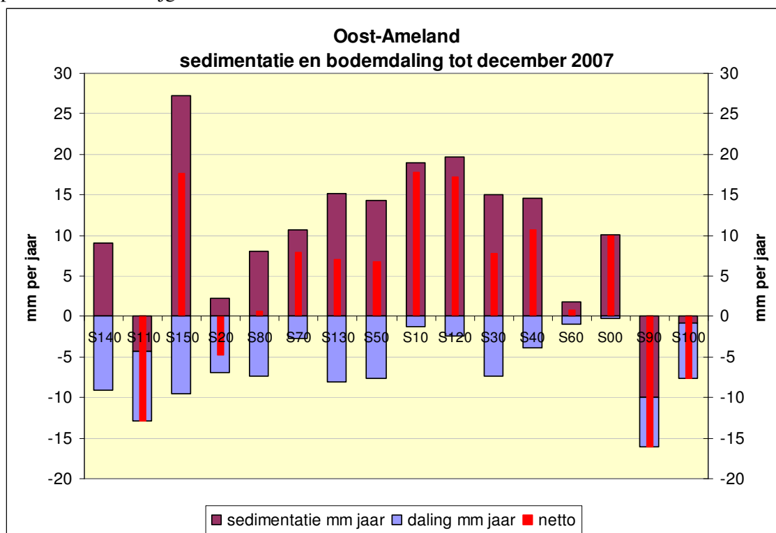
Figuur 22. Netto gemiddelde sedimentatie/erosie per jaar gedurende de gehele meetperiode per meetstation. Bijgewerkt tm december 2007.
