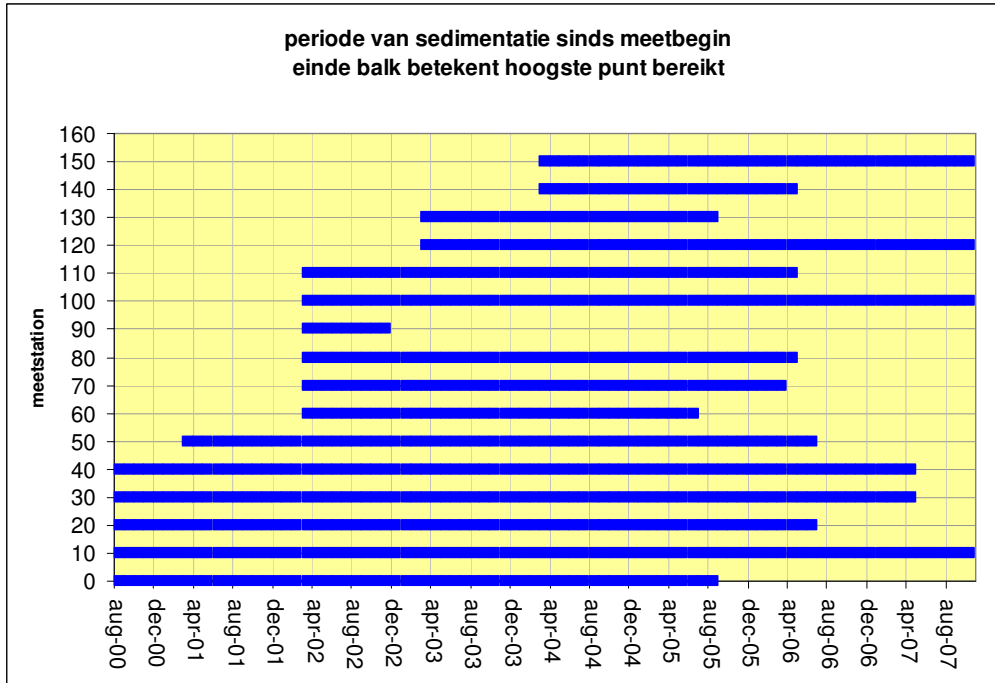
Figuur 23. Oost-Ameland. Grafische weergave van periode van begin van meting tot de hoogste gemeten waarde. Daarna volgt erosie.
