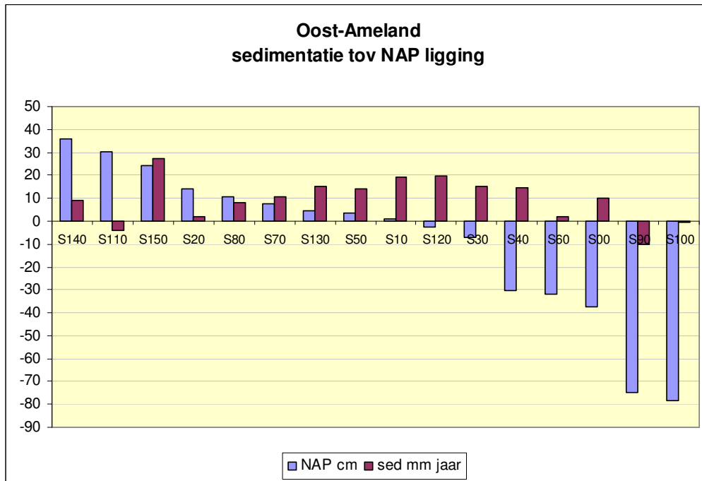
Figuur 21. Wadsedimentatie ten opzichte van hoogte ligging van de meetstations bij Oost-Ameland. Sedimentatiesnelheid in mm per jaar over de totale meetperiode. Meetperiode varieert van 3 tot 7 jaar tussen 2000 en 2007 (zie tabel 1). Meetdatum december 2007.
