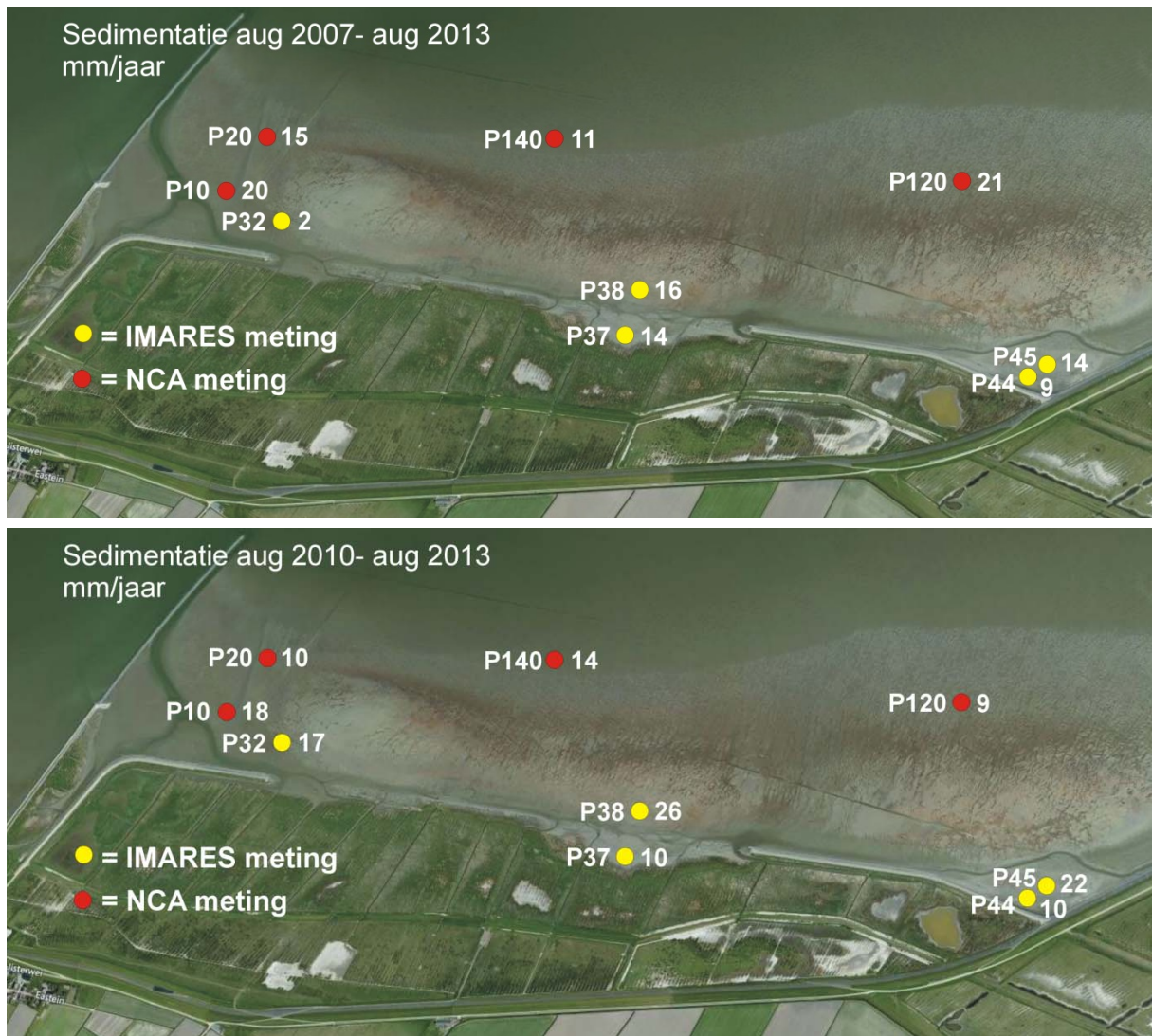
Figuur 3.4. Vergelijking van de opslibingsmetingen van NCA (rode punten) en IMARES (gele punten) op de grens van kwelder en wad bij de Peazemerlannen. Boven over periode aug 2007-aug 2013. Onder over periode aug 2010-aug 2013. De P met nummer betreft het meetpunt en het getal achter de stip de opslibing in mm/j. Figuur gemaakt door Johan Krol (NCA).
