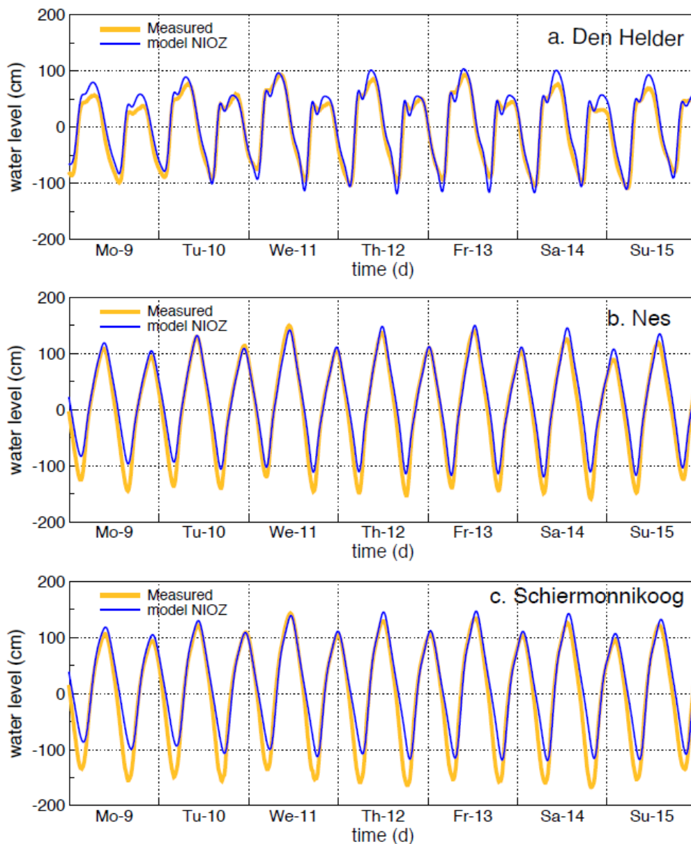
Figuur 12-3. Getijcurves voor week 32 van 2010 (9 t/m 15 augustus). De gemeten waarden zijn die van Rijkswaterstaat. De waarden voor "model NIOZ" zijn berekend met de resultaten van een hydrodynamisch model (Nauw et al. 2017).
