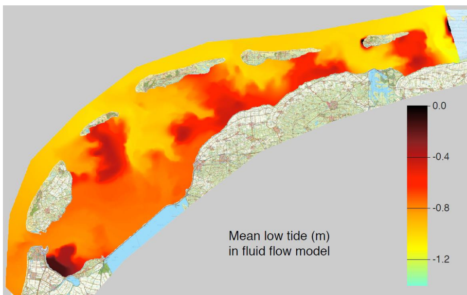
Figuur 12-2. Kaart van de gemiddelde laagwaterstand voor 2009–2011 berekend op basis van simulaties door (Nauw et al. 2017).
