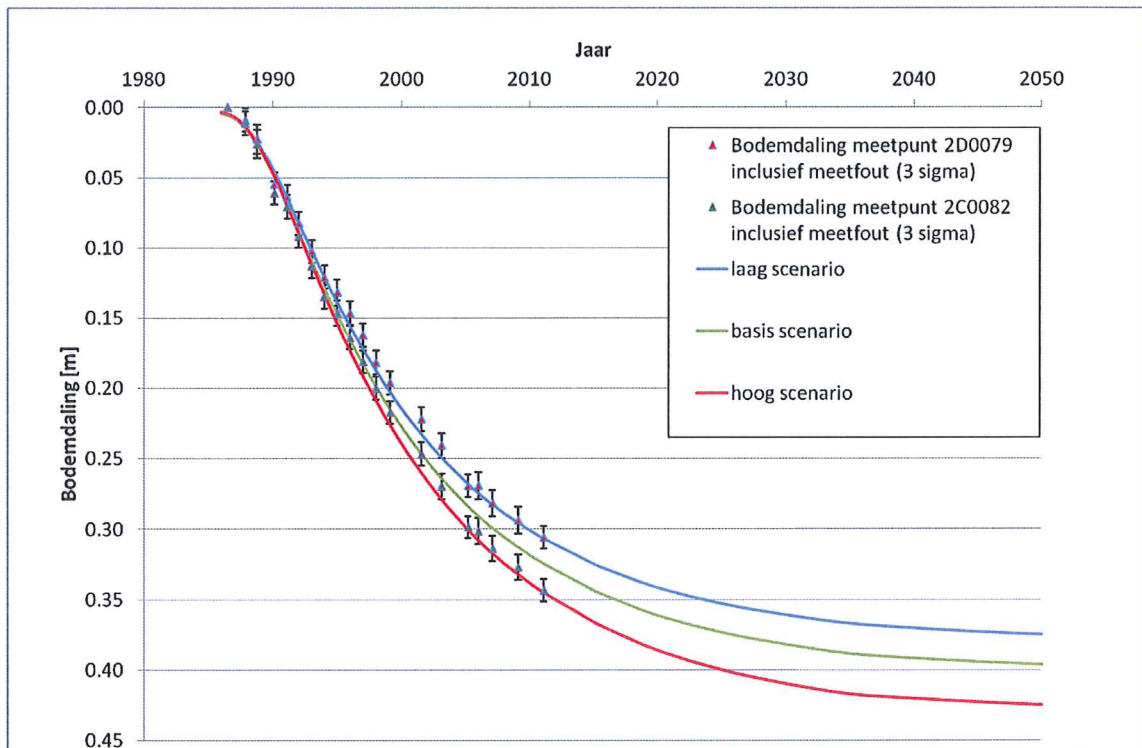
Figuur C8 Bodemdaling volgens model vergeleken met de gemeten daling op meetpunt 2D0079 en 2C0082.
