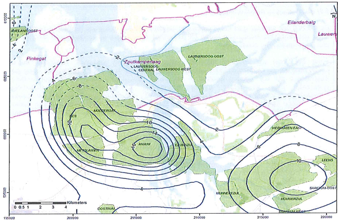
Fig. C9 Bodemdalingprognose voor 2025 van de totale bodemdaling door gaswinning uit de in dit winningsplan beschreven voorkomens in combinatie met naburige voorkomens. De contourlijnen geven de bodemdaling in cm aan.
