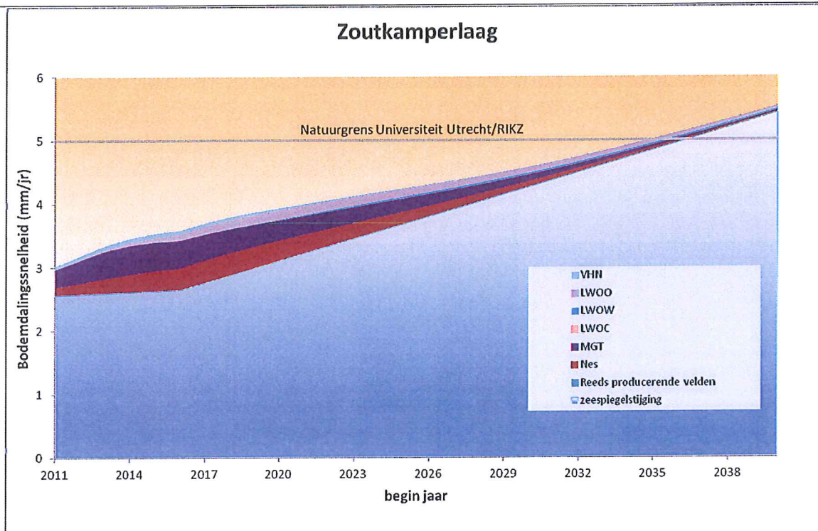
Fig. C12. Zesjaarlijks voortschrijdend gemiddelde van de bodemdalingssnelheid in het kombergingsgebied Zoutkamperlaag (mm/jaar) bij toepassing van het productieprofiel uit sectie B5.3 en de zeespiegelstijging zoals gegeven door EL&I. (geactualiseerd april 2011)
