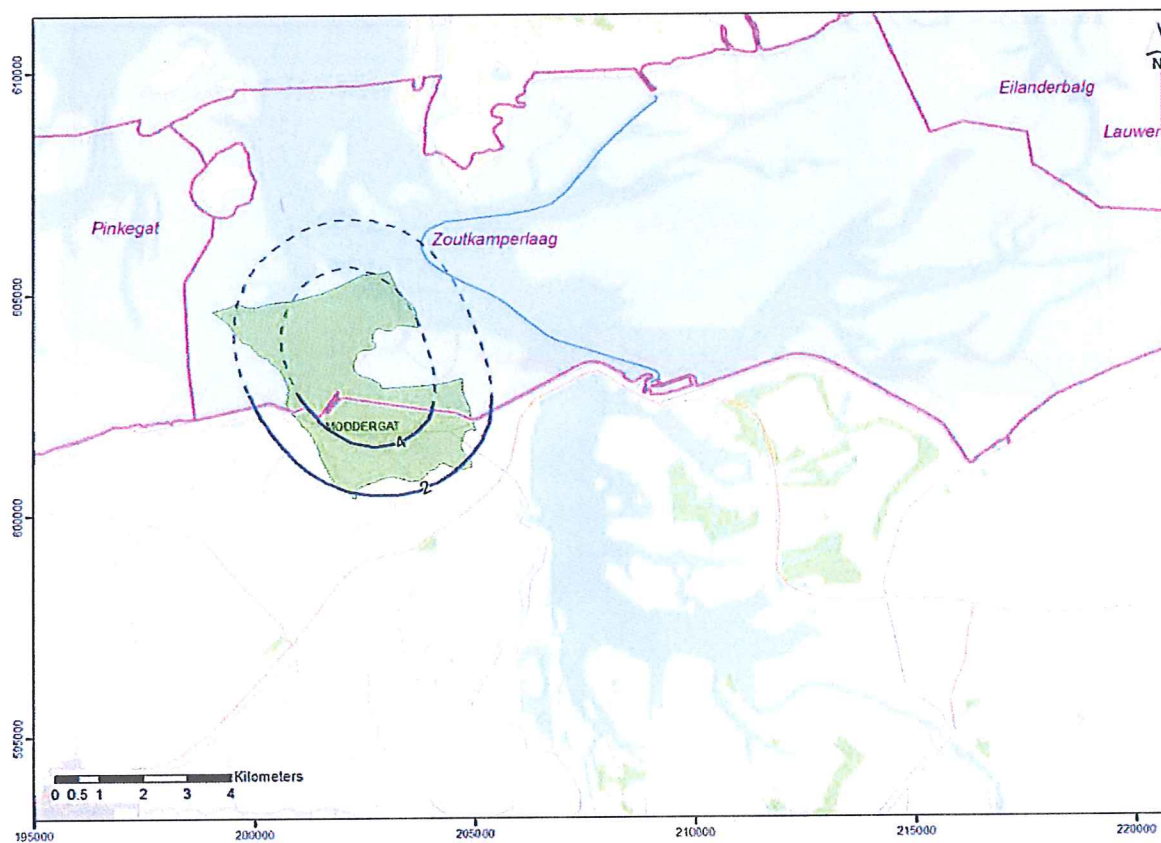
Fig. C3 Te verwachten bodemdaling in cm (2011 – 2050) veroorzaakt door de gasproductie uit het voorkomen Moddergat.
