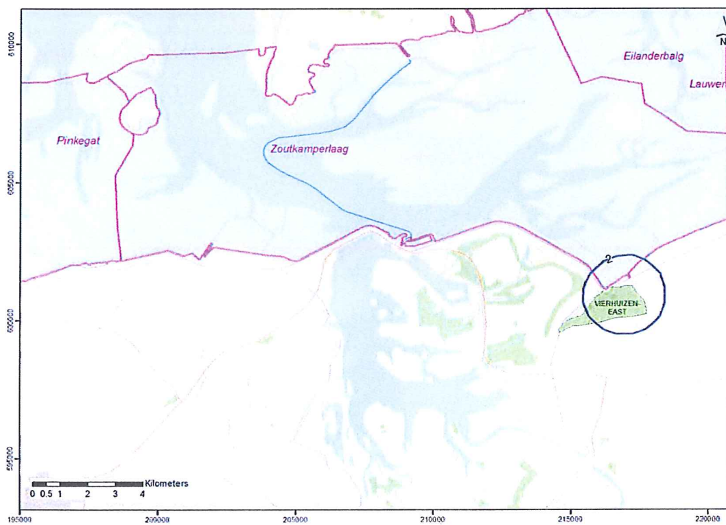
Fig. C5 Te verwachten bodemdaling in cm (2011 – 2050) veroorzaakt door de gasproductie uit het voorkomen Vierhuizen-Oost.
