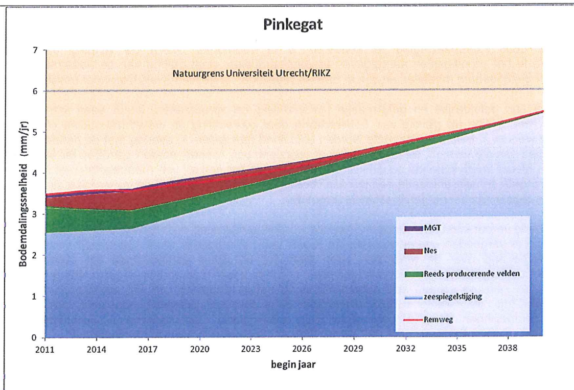
Fig. C12 Zesjaarlijks voortschrijdend gemiddelde van de bodemdalingssnelheid in het kombergingsgebied Pinkegat (mm/jaar) bij toepassing van het productieprofiel uit sectie B5.3 en de zeespiegelstijging zoals gegeven door EL&I (geactualiseerd april 2011). Tevens is de remweg bij beëindiging van de productie in 2015 getoond.
