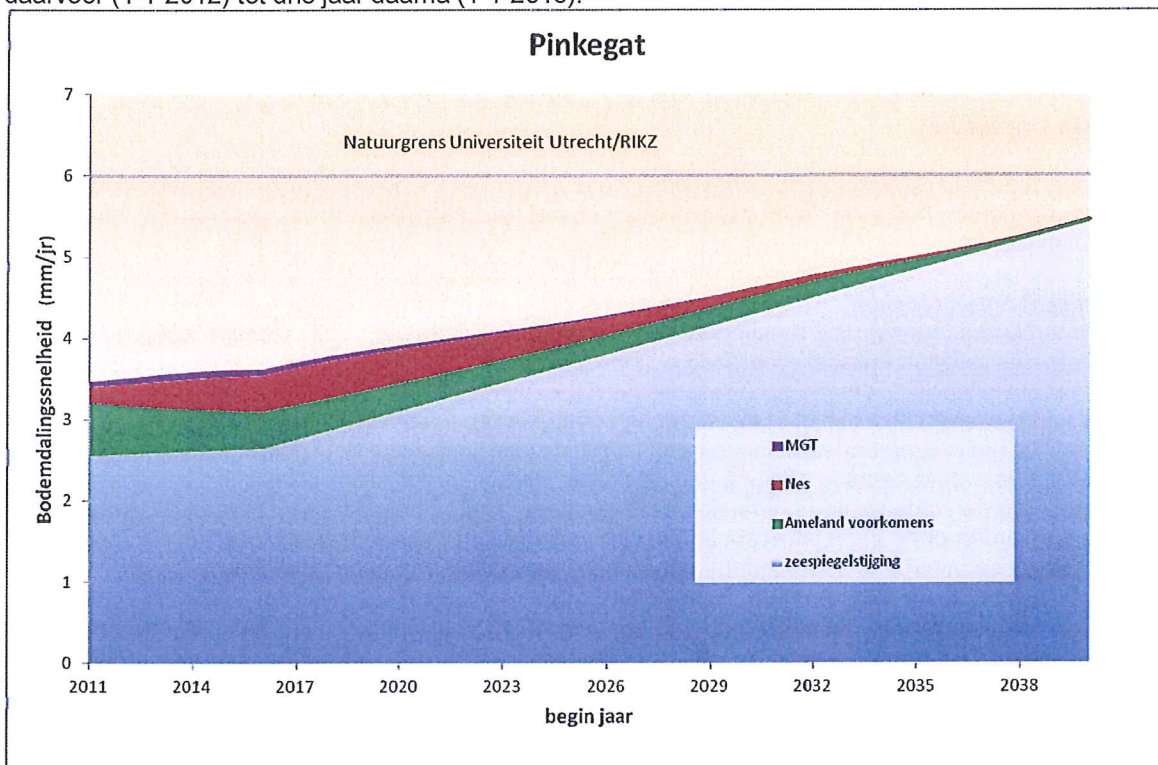
Fig. C11. Zesjaarlijks voortschrijdend gemiddelde van de bodemdalingssnelheid in het kombergingsgebied Pinkegat (mm/jaar) bij toepassing van het productieprofiel uit sectie B5.3 en de zeespiegelstijging zoals gegeven door EL&I (geactualiseerd april 2011)
