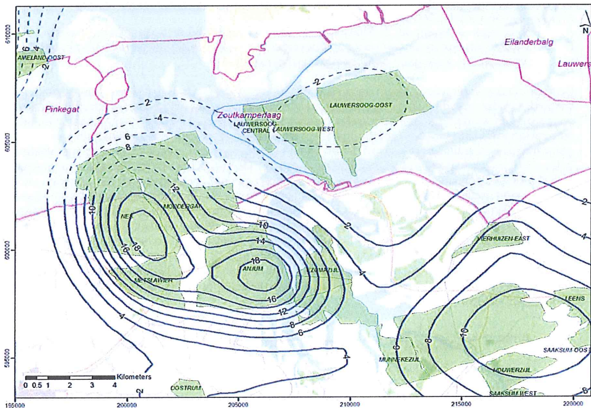
Fig. C10 Bodemdalingprognose voor 2025 van de totale bodemdaling door gaswinning uit de in dit winningsplan beschreven voorkomens in combinatie met naburige voorkomens. De contourlijnen geven de bodemdaling in cm aan.
