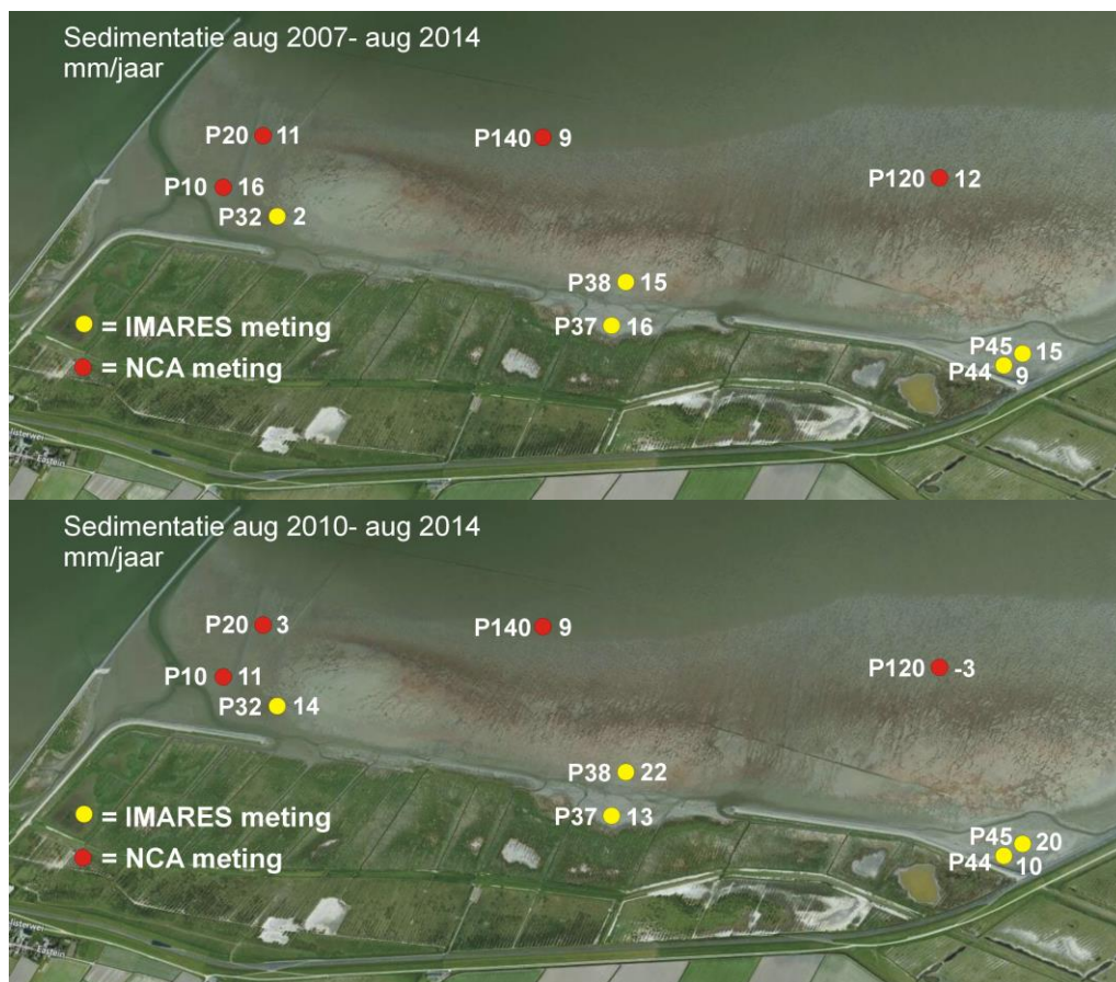
Figuur 35. Kaartbeeld met sedimentatie vergelijking van de meting van NCA en IMARES. Boven over periode aug2007-aug2014. Onder over periode aug2010-aug2014. Rechts van de gekleurde stip waarmee de locatie van het meetstation wordt aangeduid staat de sedimentatie in mm/jaar.
