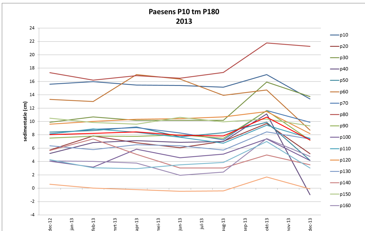
Figuur 37. Sedimentatie in 2013 van de stations P10 tm P180 in het onderzoeksgebied bij Paesens. Het effect van sterke sedimentatie op 28 oktober 2013 en sterke erosie na de storm van 6 december 2013 is op alle stations zichtbaar.
