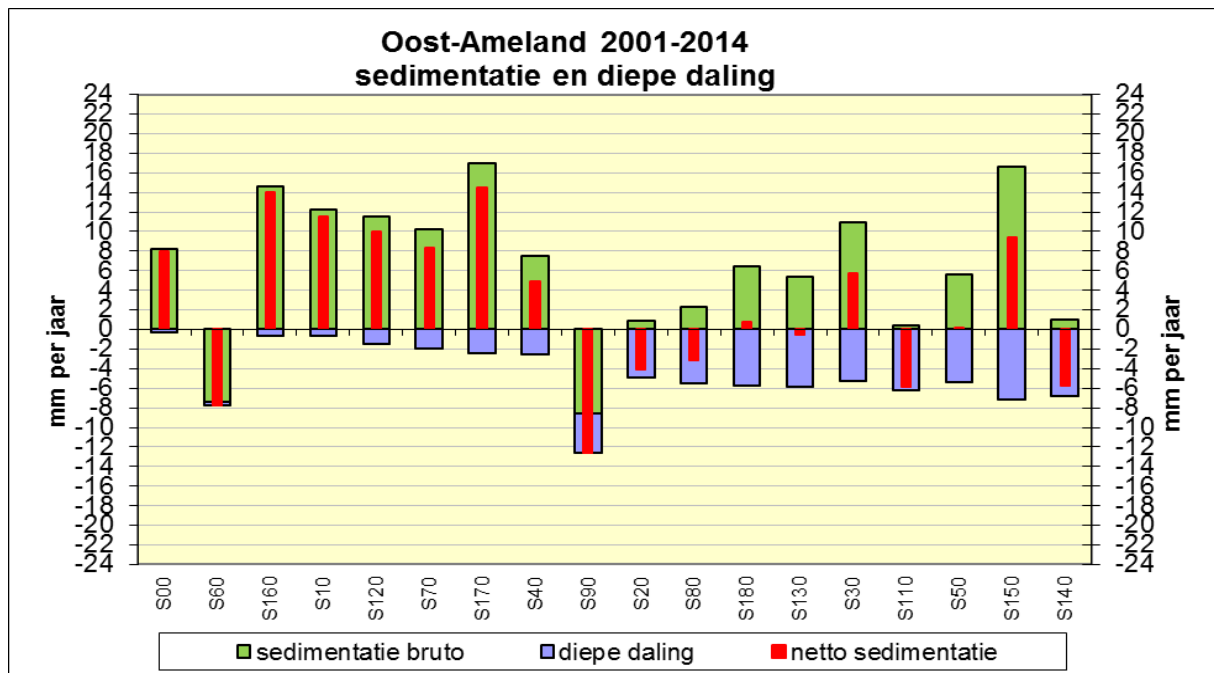
Figuur 31. Snelheid van sedimentatie en diepe bodemdaling in mm/jaar per meetstation (zie tabel 1). Diepe daling berekend over feb 2001-feb 2014. De sedimentatie aan het oppervlak is berekend tm 2014.
