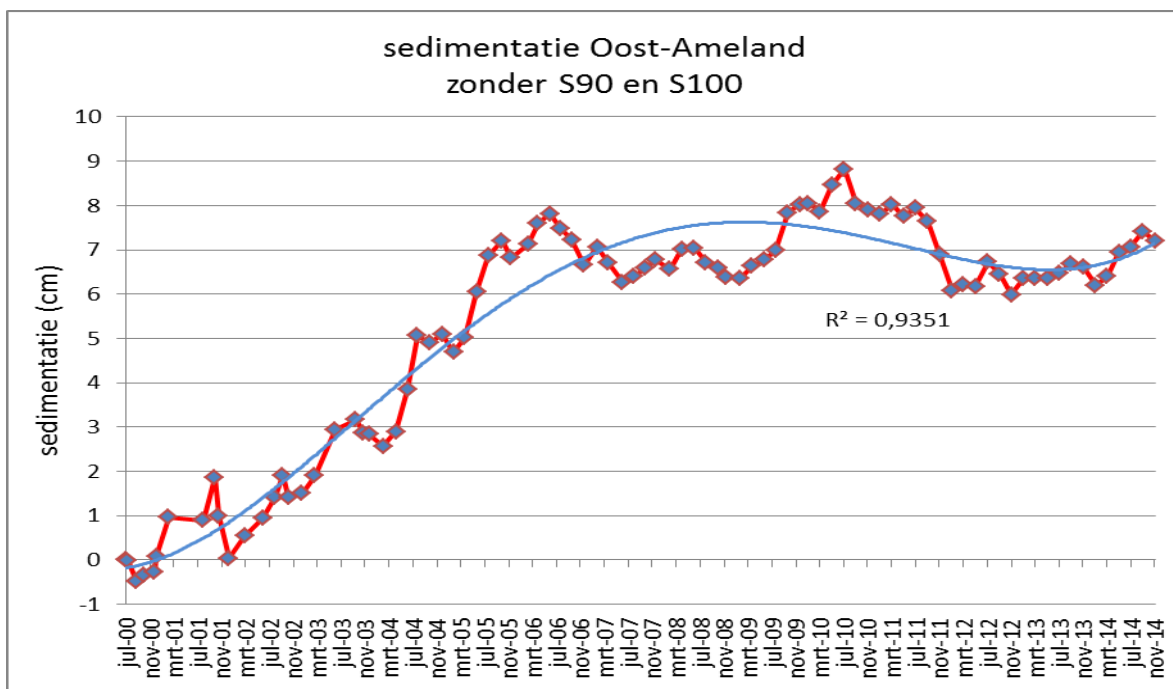
Figuur 21. Verschilmeting per keer en cumulatie van de meetstations S00 tm S180 (zonder S90 en S100) in het onderzoeksgebied Oost-Ameland.
