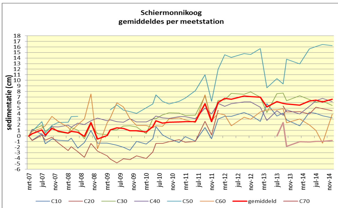
Figuur 18. Gemiddelde meetlijnen van de meetstations C10 tm C70 in het onderzoeksgebied Schiermonnikoog. Tevens is het gemiddelde van deze 7 meetlijnen genomen als weergave van de sedimentatie van het gebied waarin de meetstations liggen.
