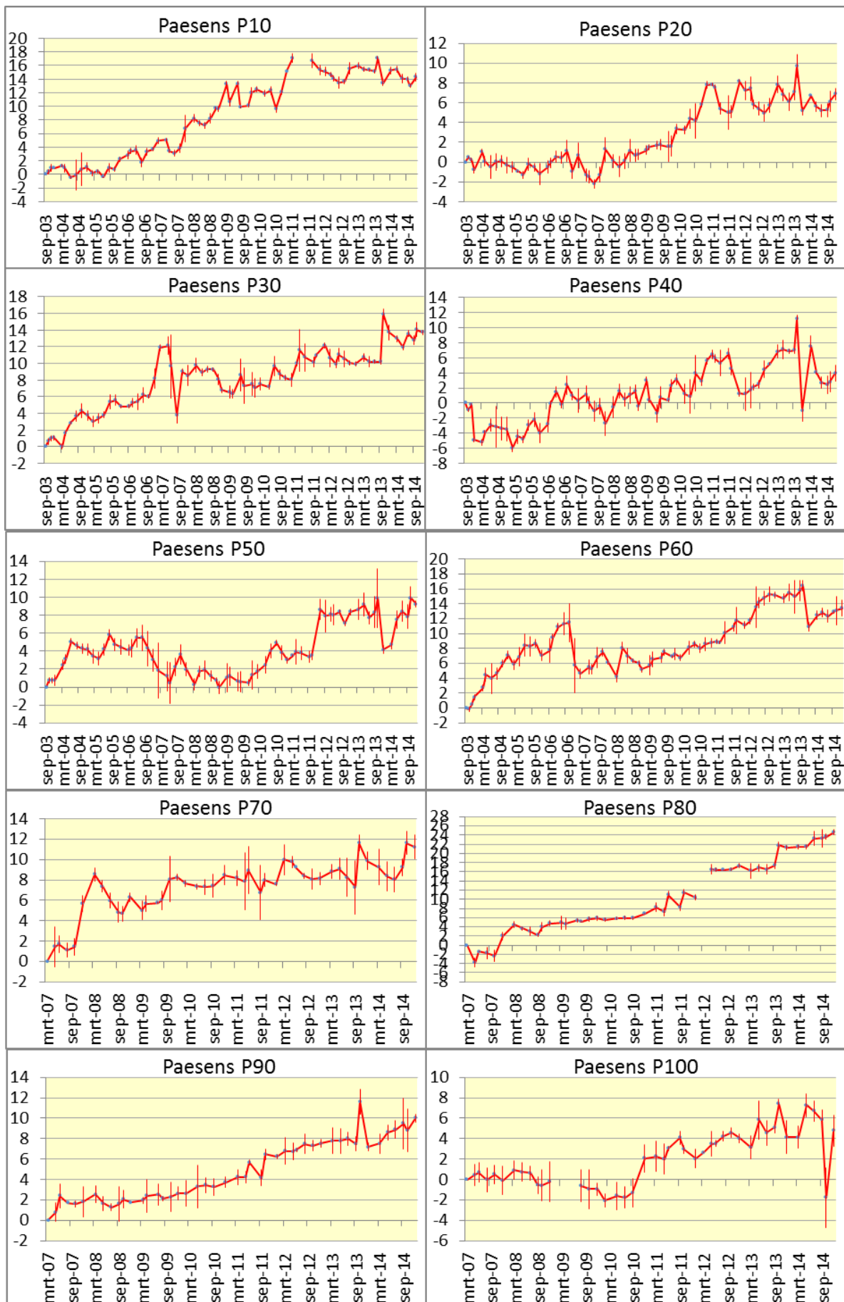
Bijlage A. Grafieken gemiddelde sedimentatie en SD van alle meetstations onderzoeksgebied Paesens bijgewerkt tm 2014. Op Y-as sedimentatie in cm.
