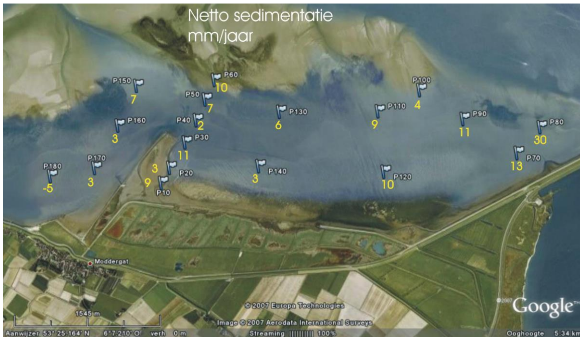
Figuur 34. Netto sedimentatie in millimeters per jaar. Sedimentatiemeting bijgewerkt tm 2014. Diepe daling berekend over periode 2007 tm 2012. Netto betekent dat de diepe daling van de sedimentatie is afgetrokken. Andere compenserende of versterkende factoren zoals zeespiegelstijging zijn niet verwerkt.
