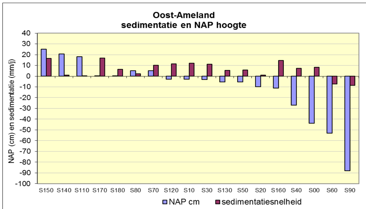
Figuur 27. Wadsedimentatie ten opzichte van hoogteligging van de meetstations bij Oost-Ameland. Sedimentatiesnelheid in mm per jaar over de totale meetperiode. Meetperiode van de meetstations varieert van 8 tot 14 jaar tussen 2000 en 2014 (zie tabel 2). Meetdatum sedimentatie is in december 2014. Een uitzondering is S100, dit station is door geulvorming in 2009 verloren gegaan.
