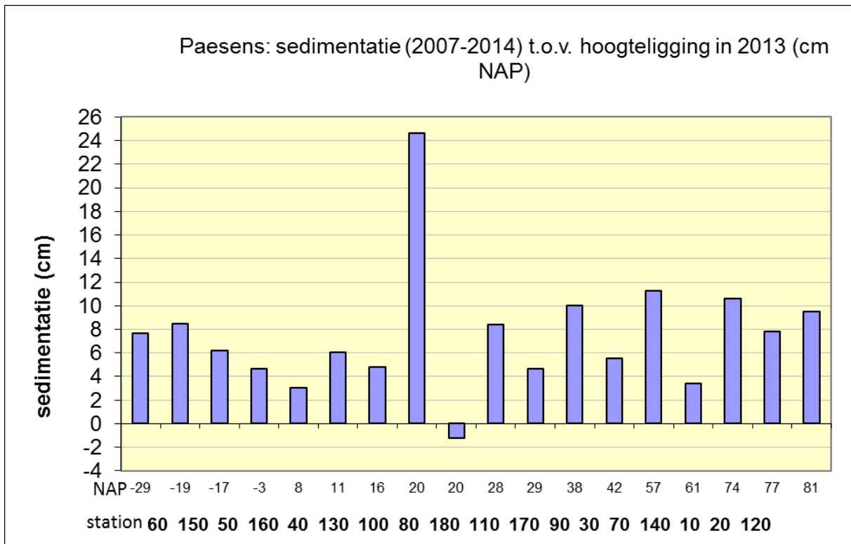
Figuur 29. Sedimentatie P10 – P180 in relatie tot de hoogteligging.
