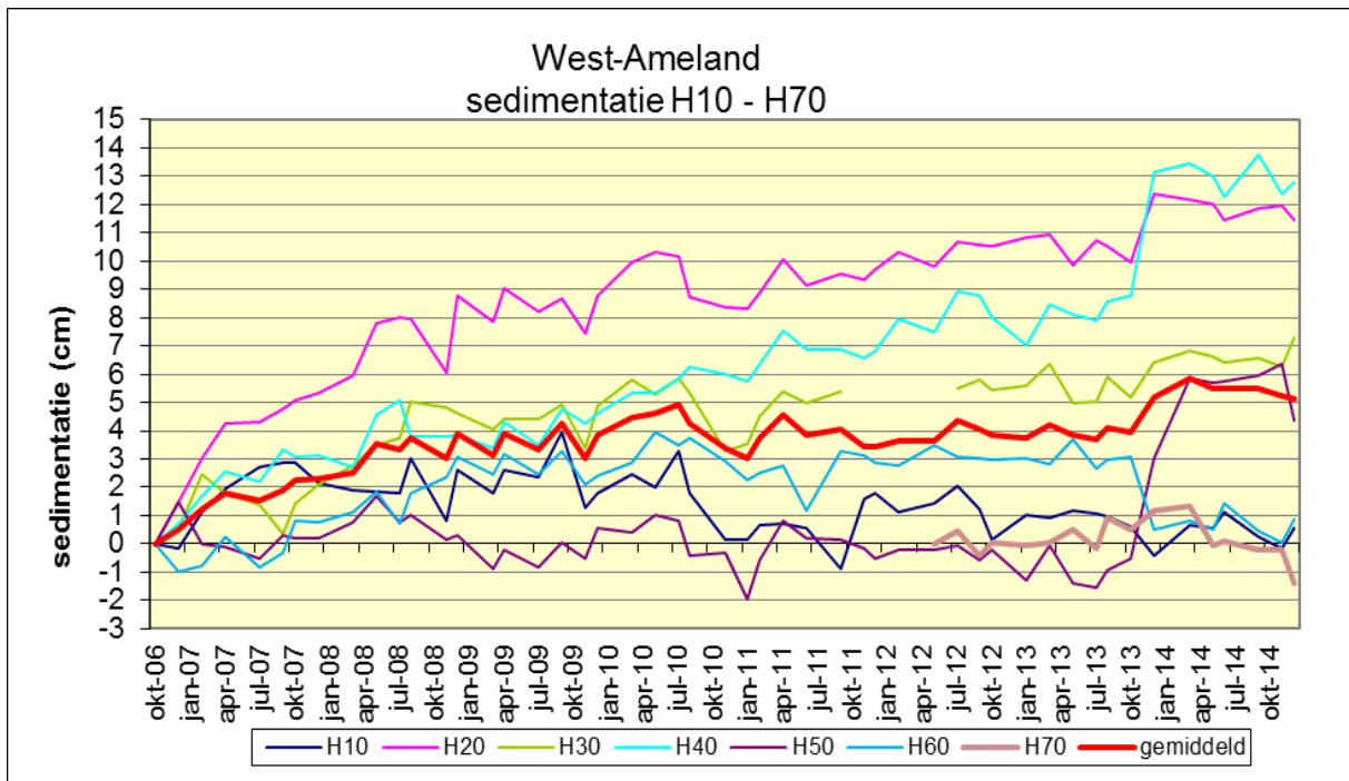
Figuur 22. Gemiddelde meetlijnen van de meetstations H10 tm H60 in het onderzoeksgebied West-Ameland.
