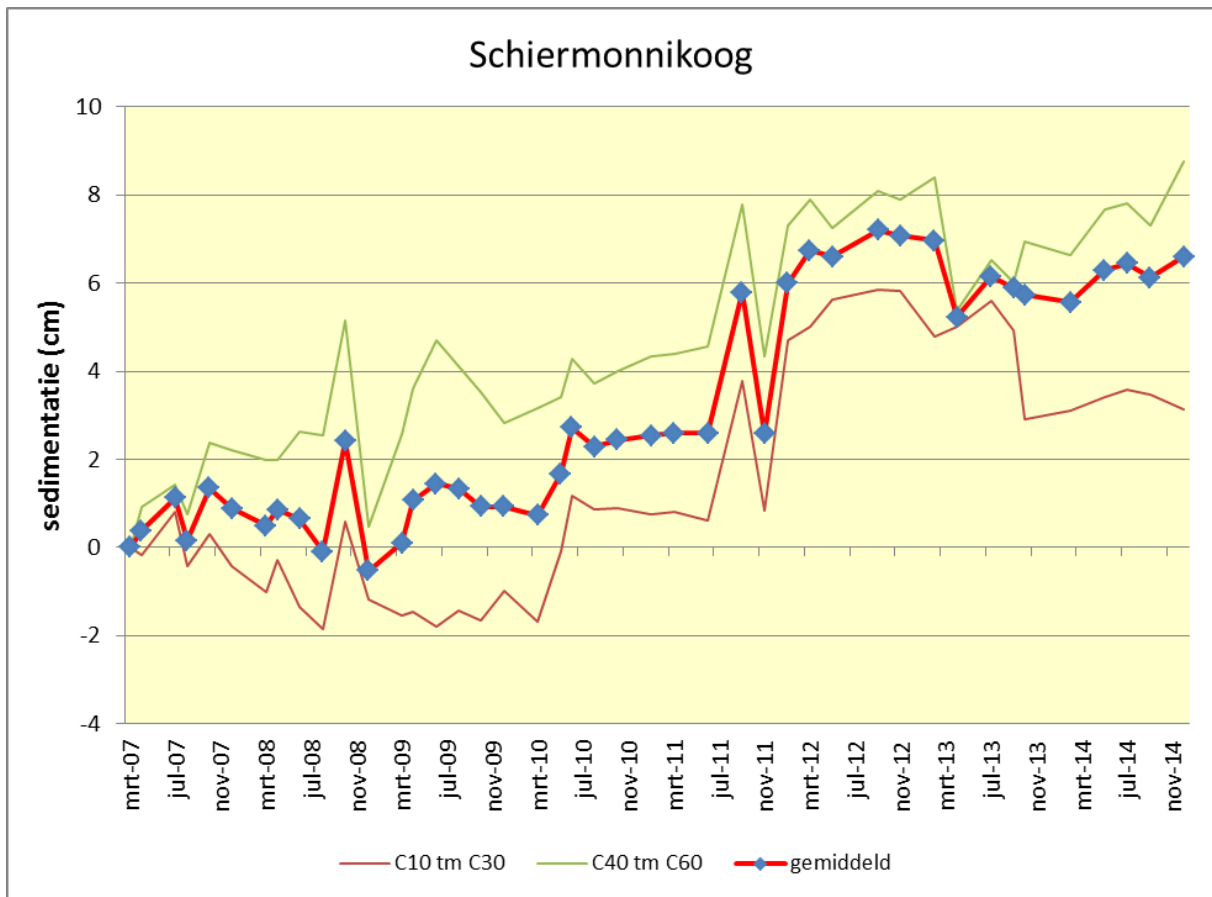
Figuur 19. Gemiddelde van de gebieden C10 – C30 en C70 (oost) en C40 – C60 (west) en het overall gemiddelde van de meetstations C10 tm C70 in het onderzoeksgebied Schiermonnikoog.
