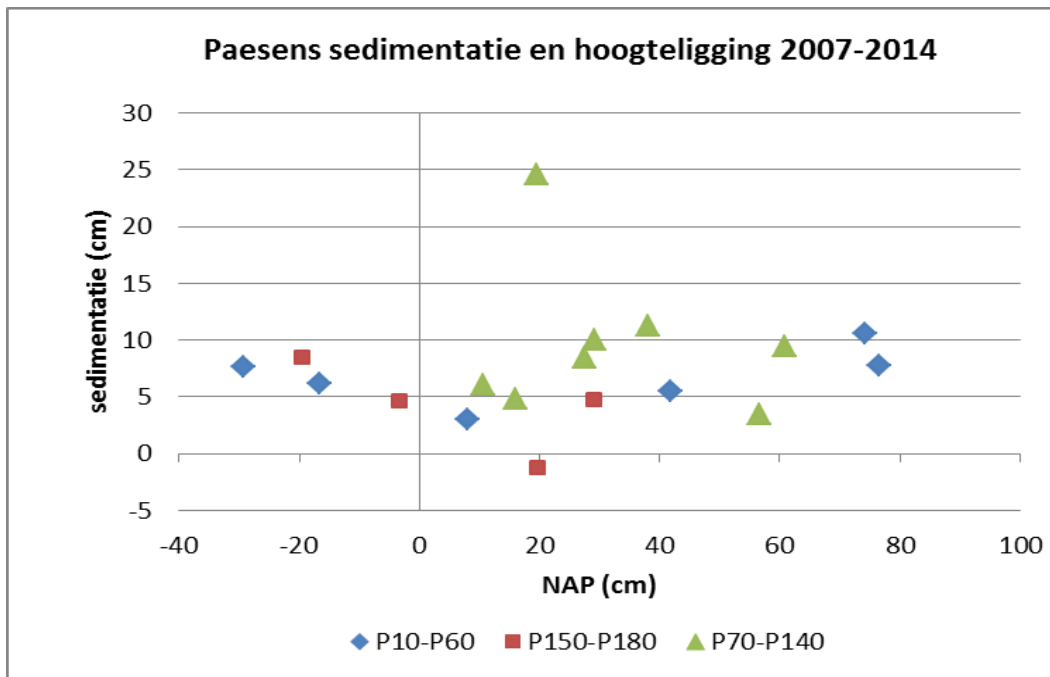
Figuur 30. Hoogteligging en sedimentatie van meetstations bij Paesens in de periode 2007-2014.
