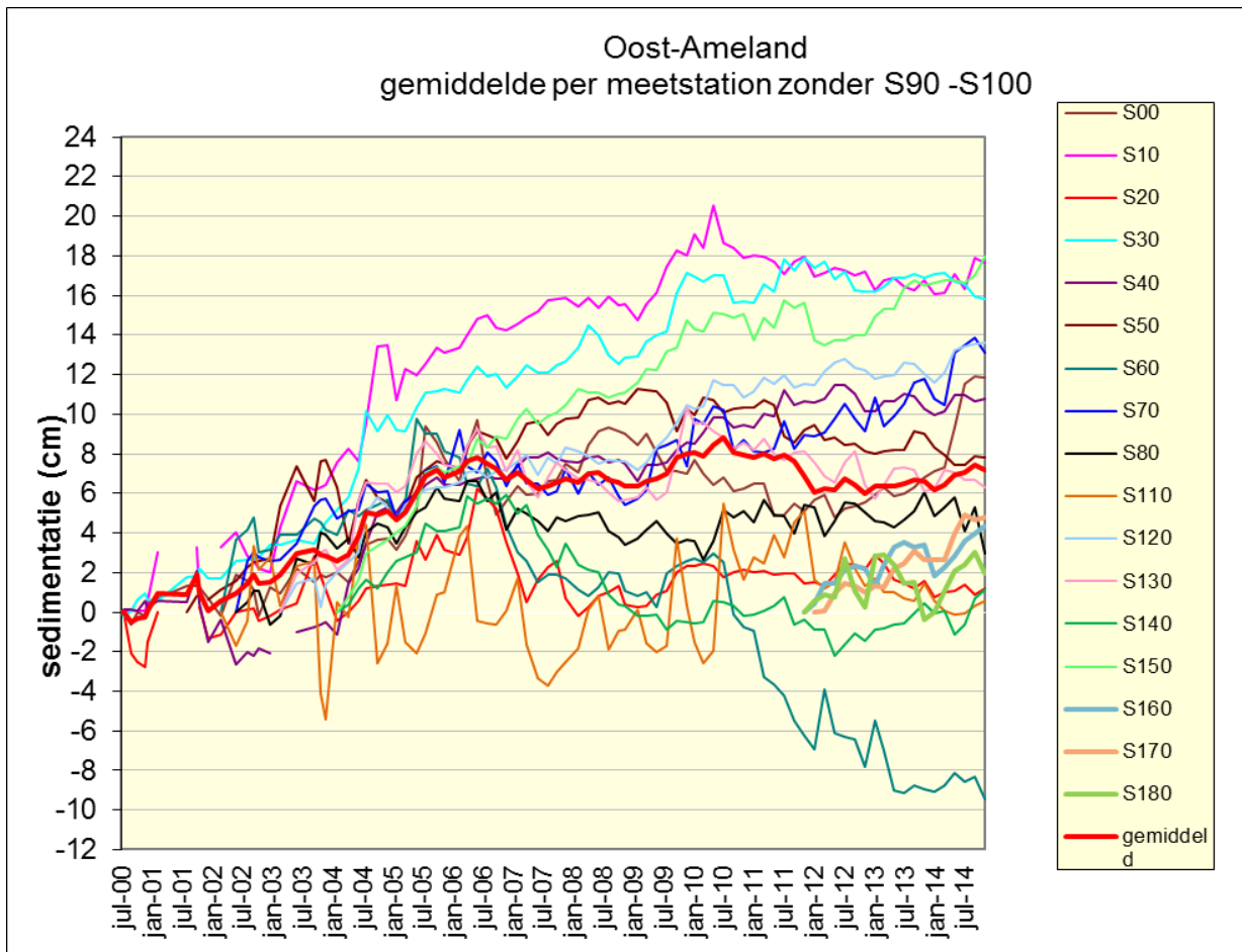
Figuur 20. Gemiddelde meetlijnen van de meetstations S00 tm S80 en S110 tm S180 in het onderzoeksgebied Oost-Ameland. De stations S160 tm S180 starten in 2012. Station S90 en S100 zijn weggelaten. S100 is in 2009 verloren gegaan en S90 is een geulwandstation en niet representatief voor plaats sedimentatie..
